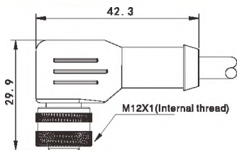
M12 Right angle
