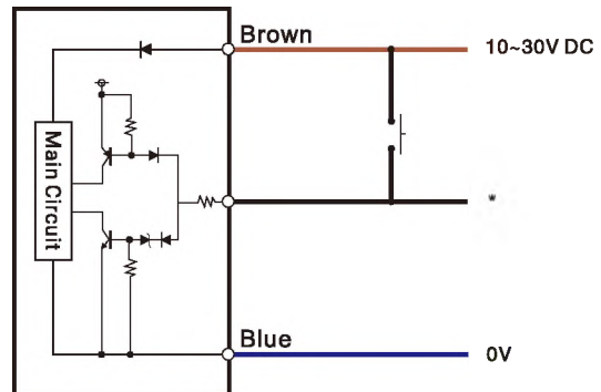
PNP output
